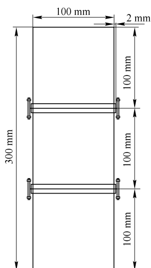
图 1 盛料器的形状与尺寸
