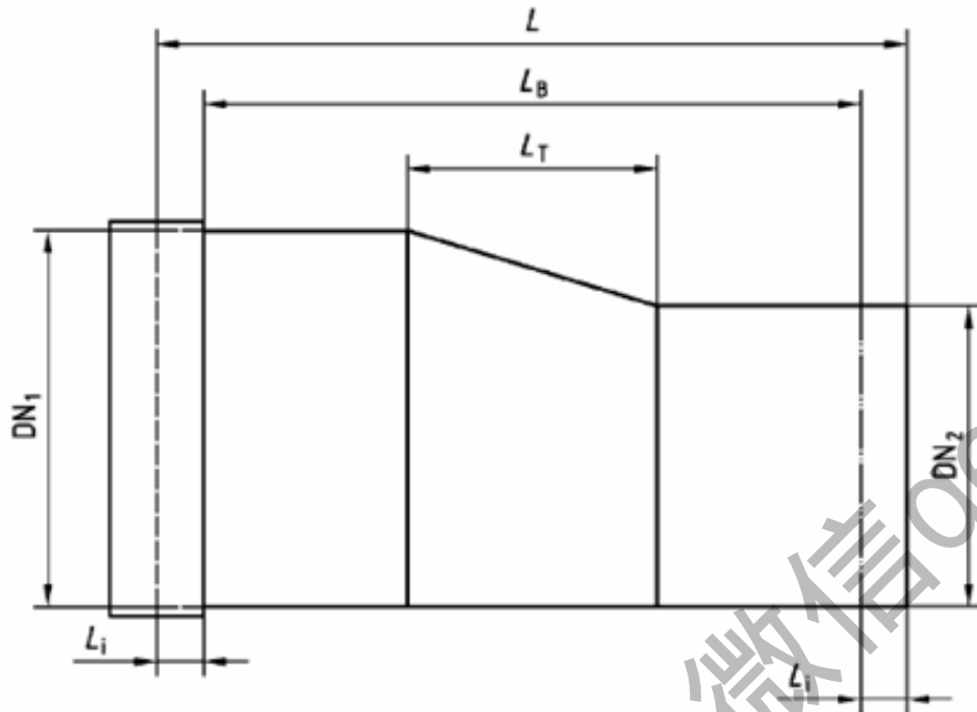
b) 偏心变径管
