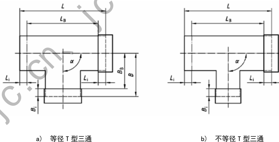
图 E.3 典型的三通
