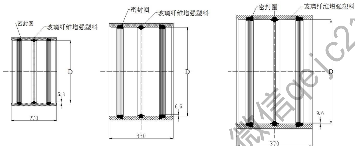
图 D.2 分体橡胶密封圈套筒接头
