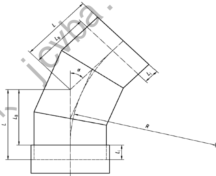
图 E.1 典型的模制弯头
