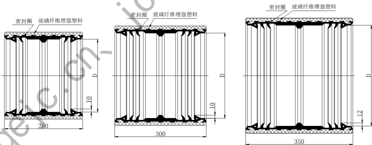
图 D.1 整体橡胶密封圈套筒接头
