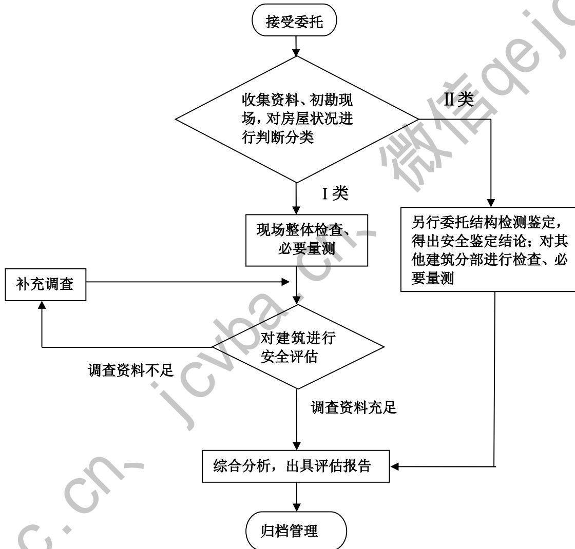
图 3.1.3 房屋建筑安全评估工作程序图
