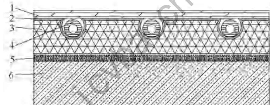
图 A-1 与供暖房间相邻的装配式地面辐射供暖供冷地面构造(一)
