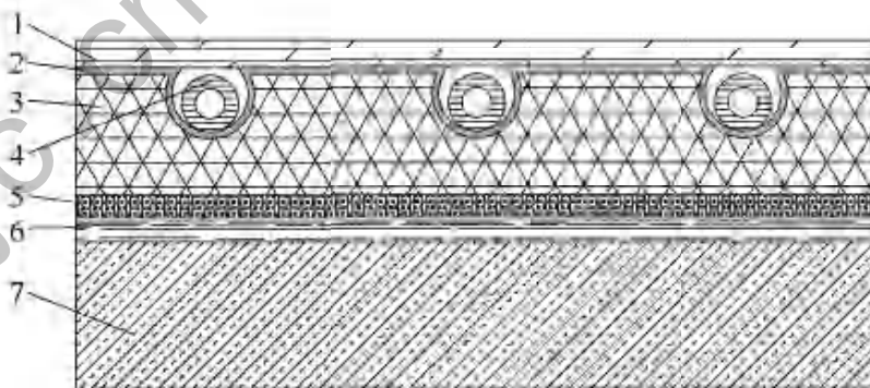
图 A-5 与土壤相邻的装配式地面辐射供暖供冷地面构造(一)
