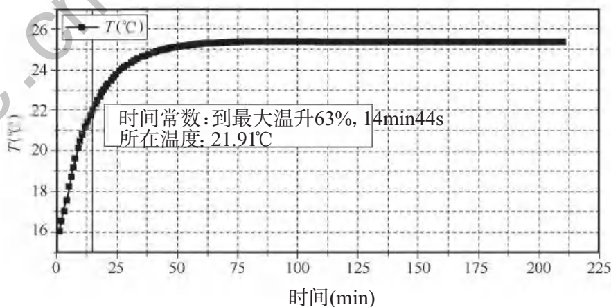
(b) 系统总变化幅度的63%
