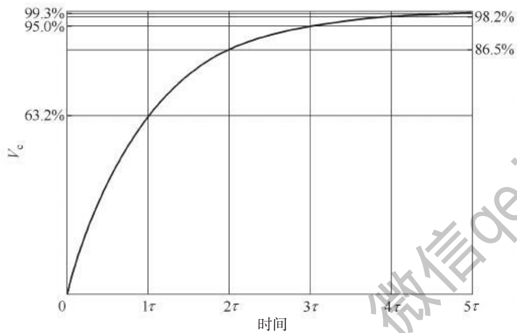
图1 不同变化幅度所消耗的时间
