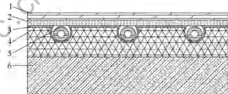
图 A-2 与供暖房间相邻的装配式地面辐射供暖供冷地面构造(二)
