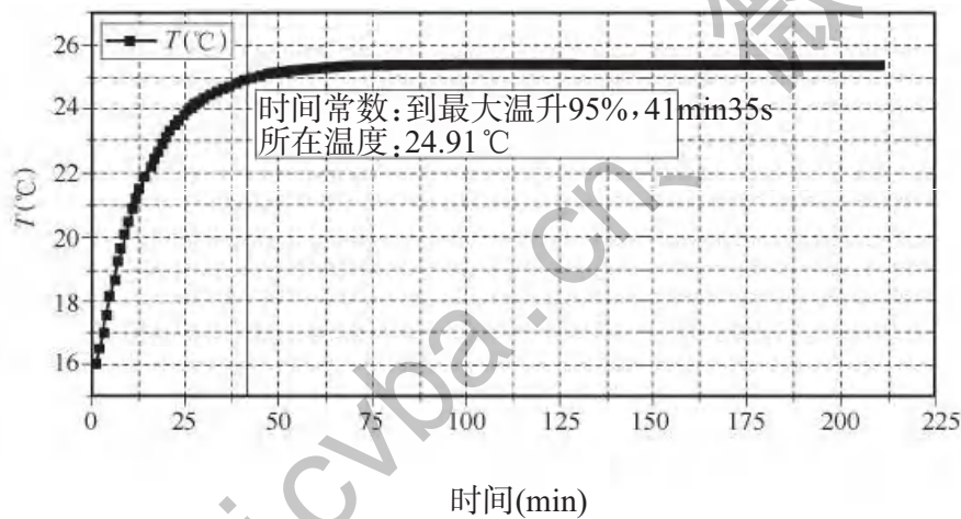
(a) 系统总变化幅度的95%
