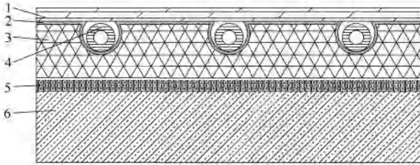
图 A-4 与室外空气或不供暖房间相邻的装配式地面辐射 供暖供冷地面构造(二)
