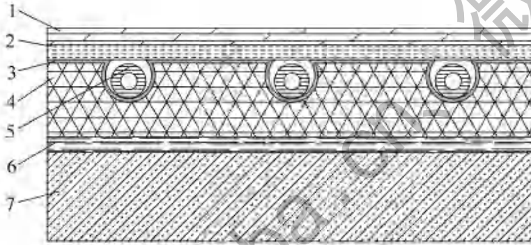
图 A-4 与室外空气或不供暖房间相邻的装配式地面辐射 供暖供冷地面构造(二)
